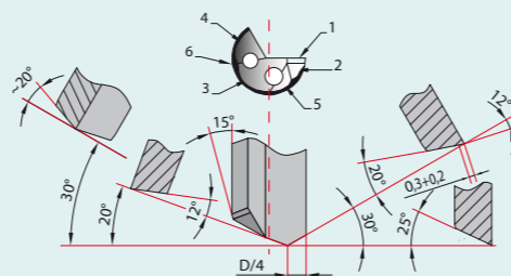
Стандартная заточка для однолезвийного сверла с D = 5 - 30 мм
