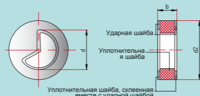
Уплотнительная шайба TBN 5404
