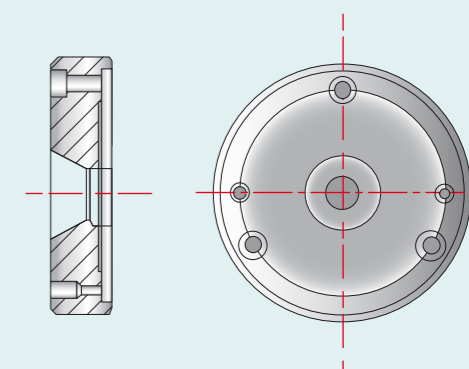
Зажимный конус
