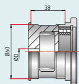
Герметичный корпус 100700-7101-01
