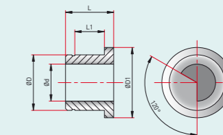
Фасонная люнетная втулка
