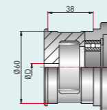
Герметичный корпус 302200-7101-01
