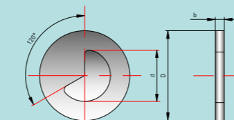
Уплотнительная шайба TBN 5416
