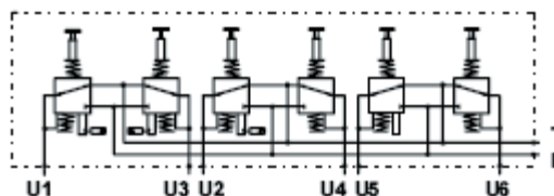
Схема подключения
